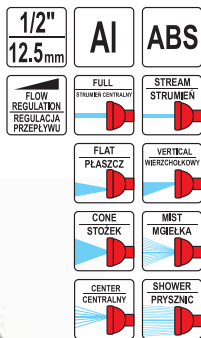
YATO size / rozmiar YT-8960 1/2" / 12.5 mm 12/48
