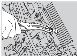
For engine air pipe Do przewodów powietrznych listwy wtryskowej
